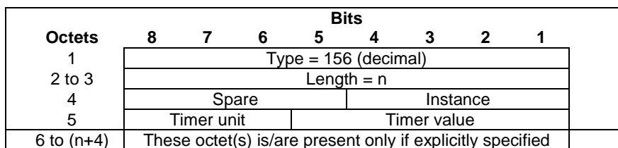
Figure 8.87-1: EPC Timer
