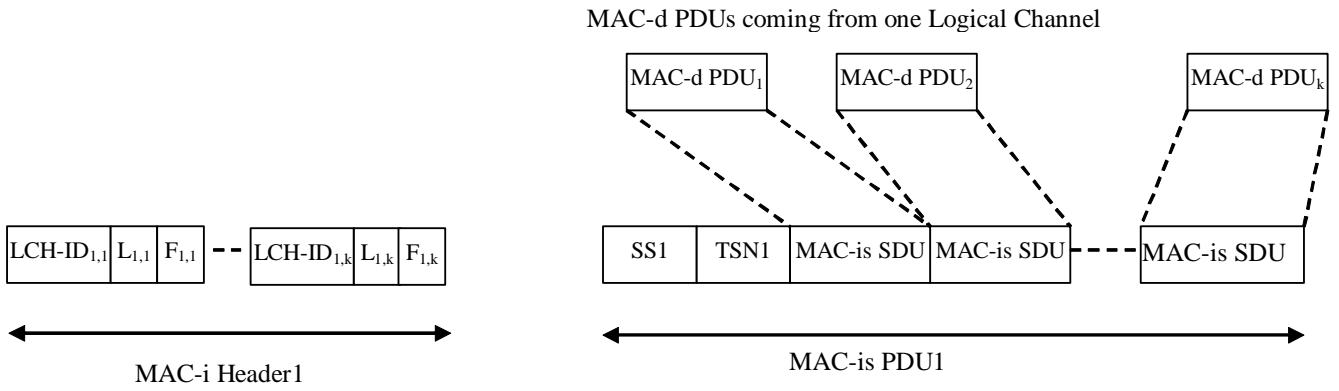
Figure 9.1.5-3 MAC-is PDU.
