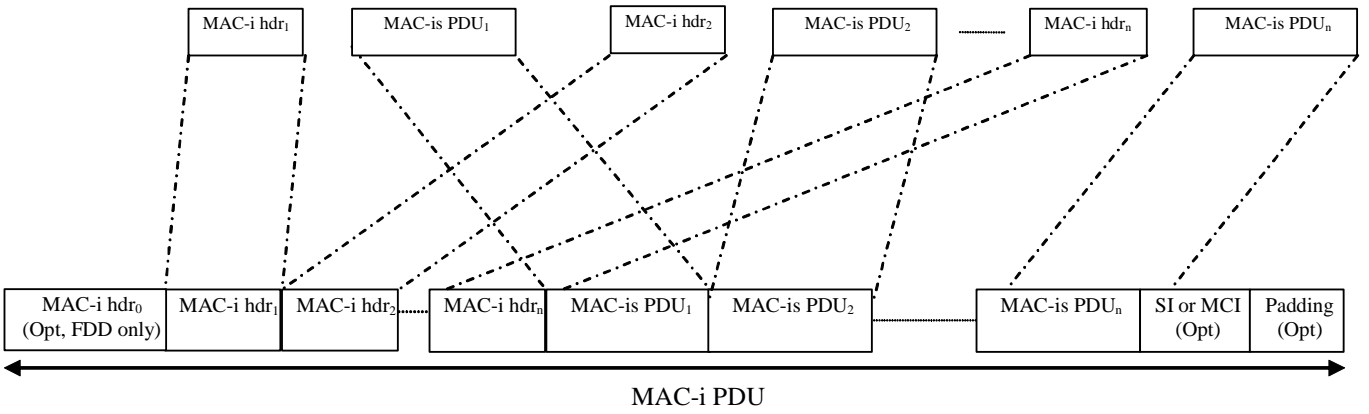
Figure 9.1.5-4a: MAC-i PDU.
