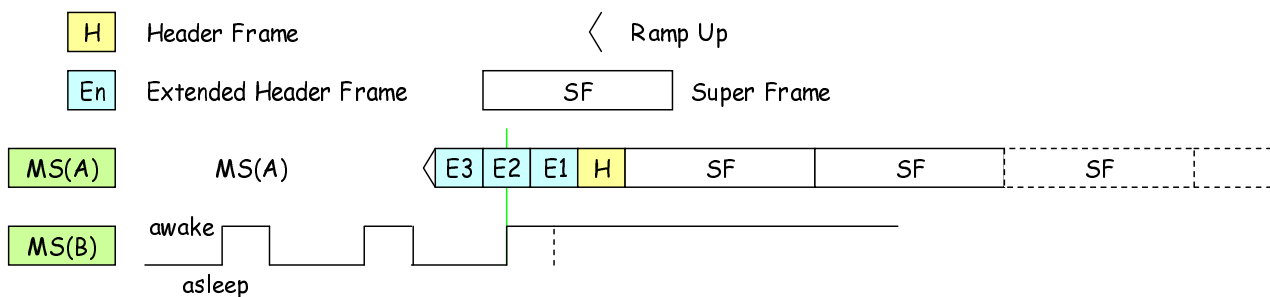
Figure 10.10 : Powersave Example
