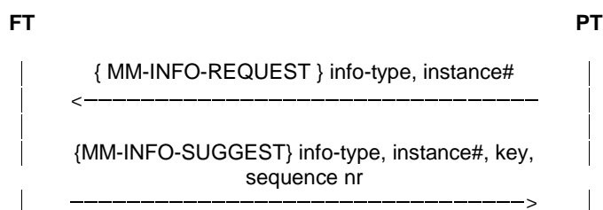
Figure 6.1b: PT parameter retrieval procedure
