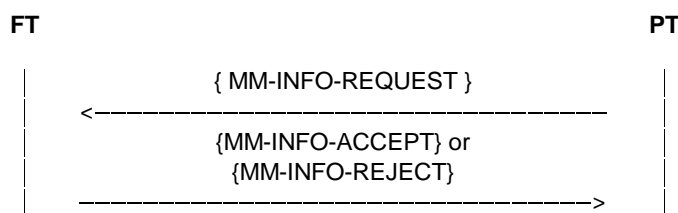
Figure 124: PT parameter retrieval procedure
