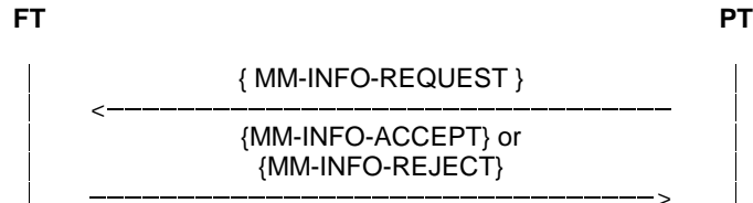
Figure 124: PT parameter retrieval procedure
