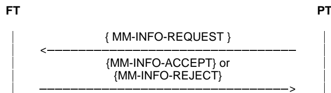
Figure 124: PT parameter retrieval procedure
