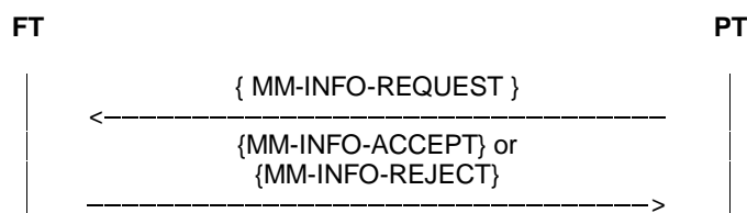
Figure 124: PT parameter retrieval procedure
