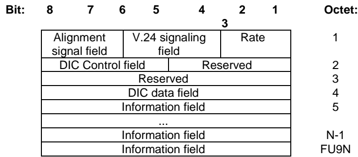
Figure 11.11.1.1.1.1: Frame Format Type FU9
