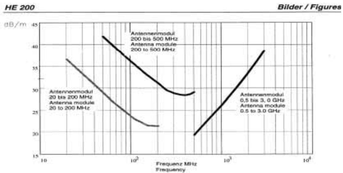
Bild 2a Antennenfaktor, Passiv-Betrieb Fig. 2a Antenna factor, passive mode
